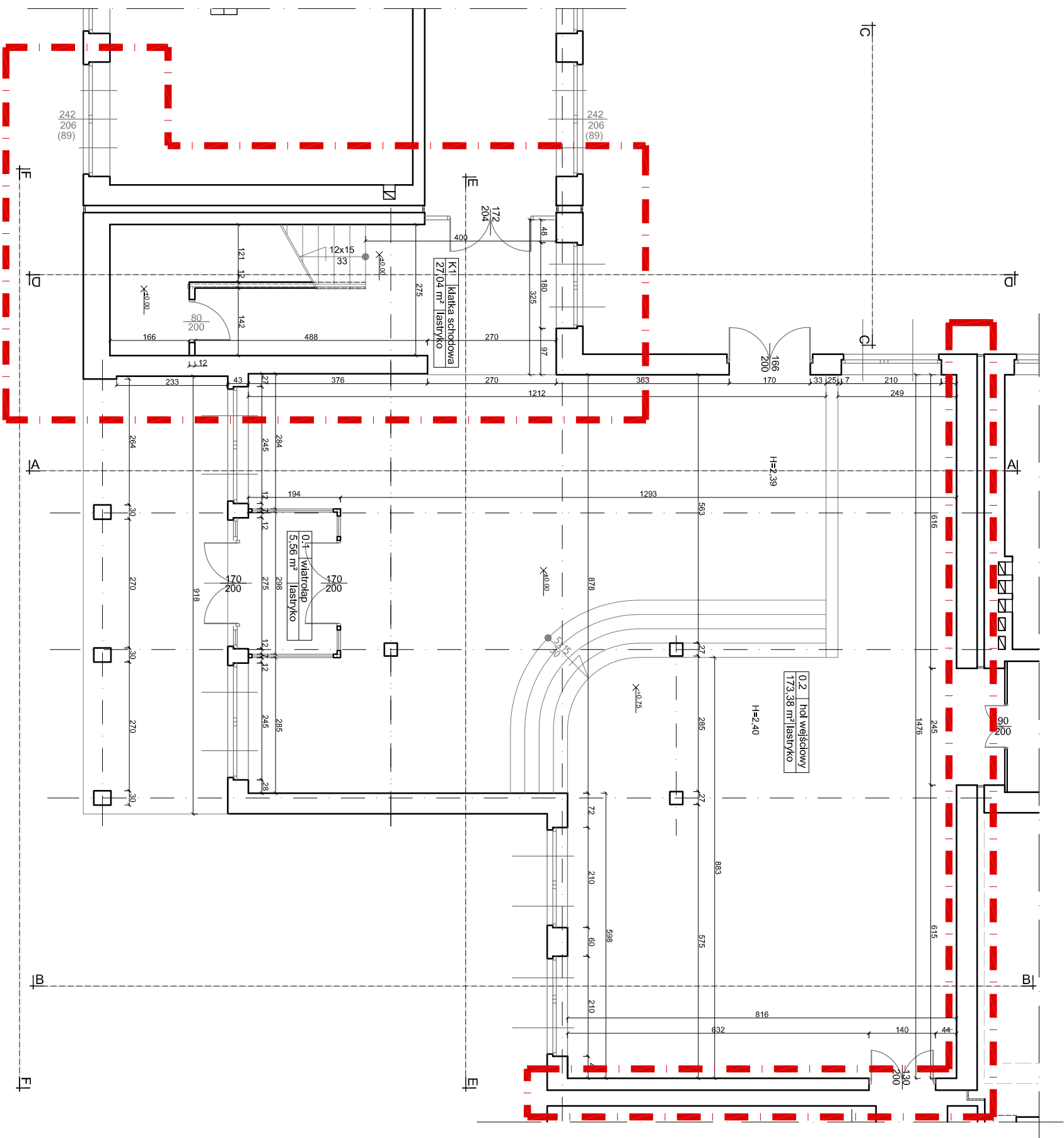
rzut parteru
